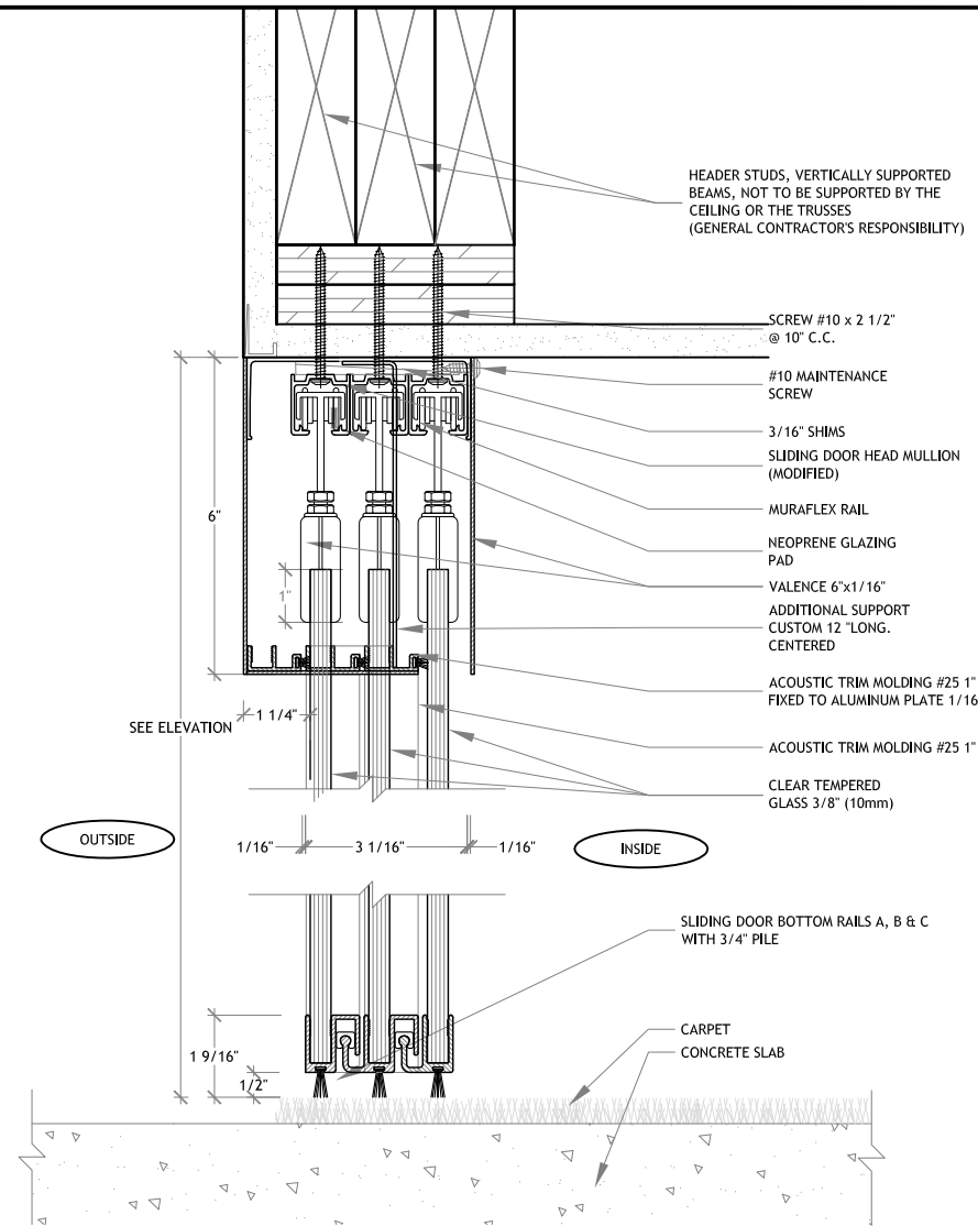
DETAIL A-A
